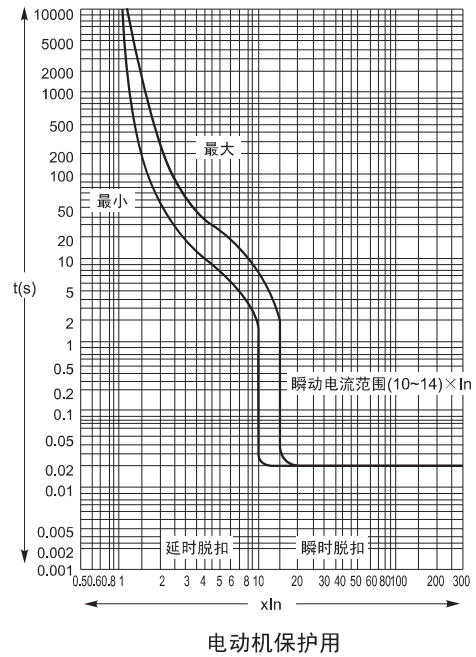
CFM1LE-400时间/电流特性曲线
