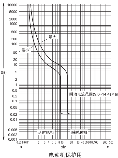
CFM1LE-250时间/电流特性曲线
