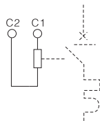
分励脱扣器+辅助开关
