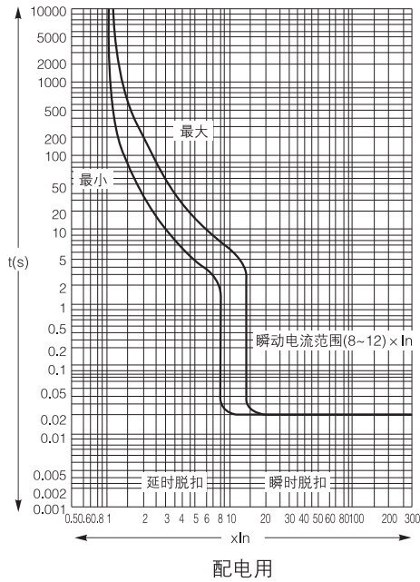
CFM1sLE-(100)125时间/电流特性曲线
