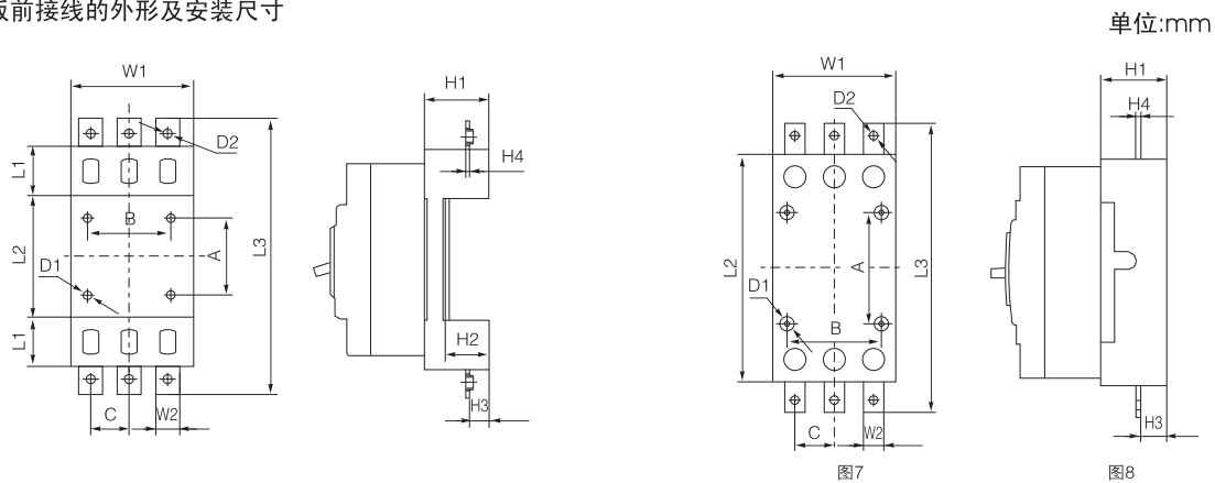
CFM1sLE-(100)125、(225)250、630、800插入式板前接线外形图
