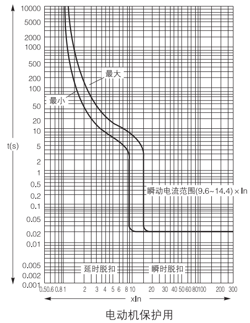
CFM1sLE-(225)250时间/电流特性曲线
