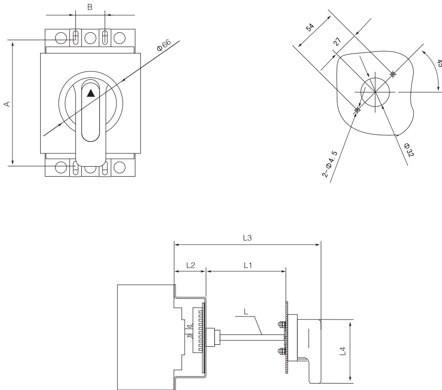
手操作机构安装示意图见图9
