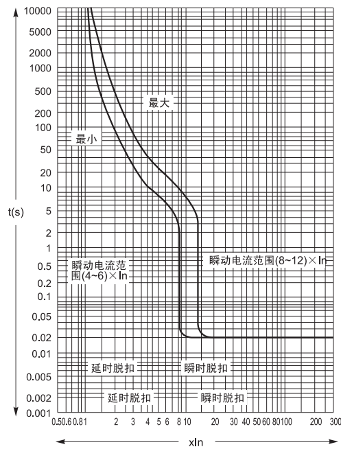
CFM1sLE-630、800时间/电流特性曲线(配电)
