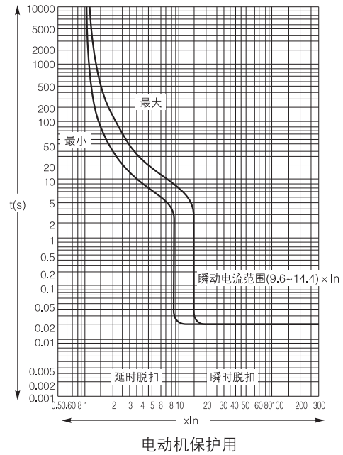
CFM1sLE-(100)125时间/电流特性曲线
