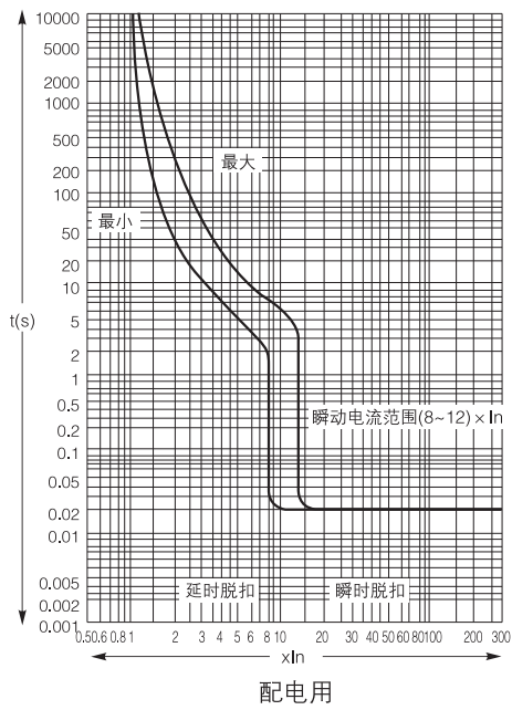
CFM1sLE-(225)250时间/电流特性曲线
