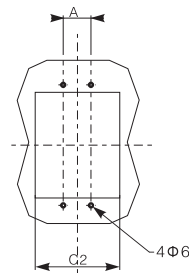
• CFM5E-400/630 3P
