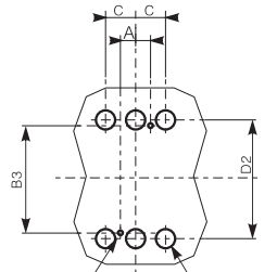
• CFM5E-100~250 2/3P
