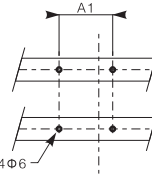
• CFM5E-100~250 4P
