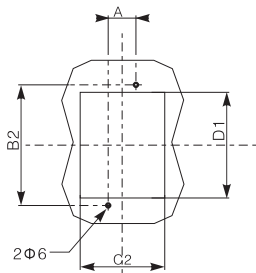
• CFM5E-100~250 2/3P
