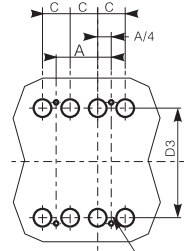
• CFM5E-100~250 4P
