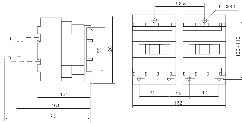
图4 CFC2-80~95N可逆接触器外形及安装尺寸
