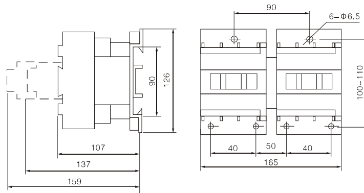
图3 CFC2-40~63N可逆接触器外形及安装尺寸
