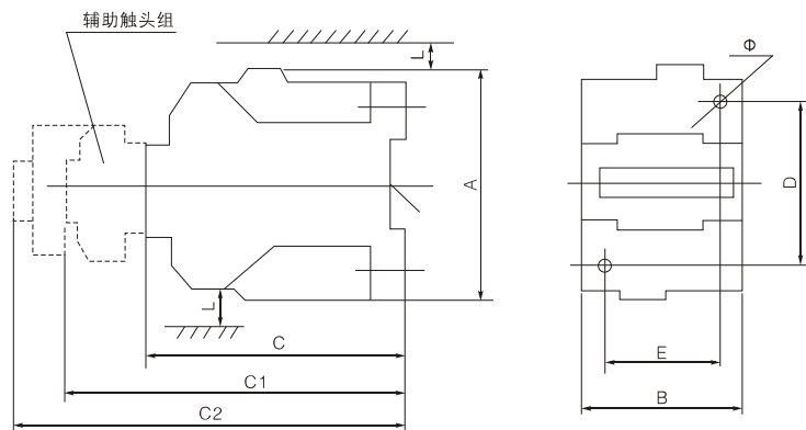
图1 CFC2系列交流接触器的外形及安装尺寸图
